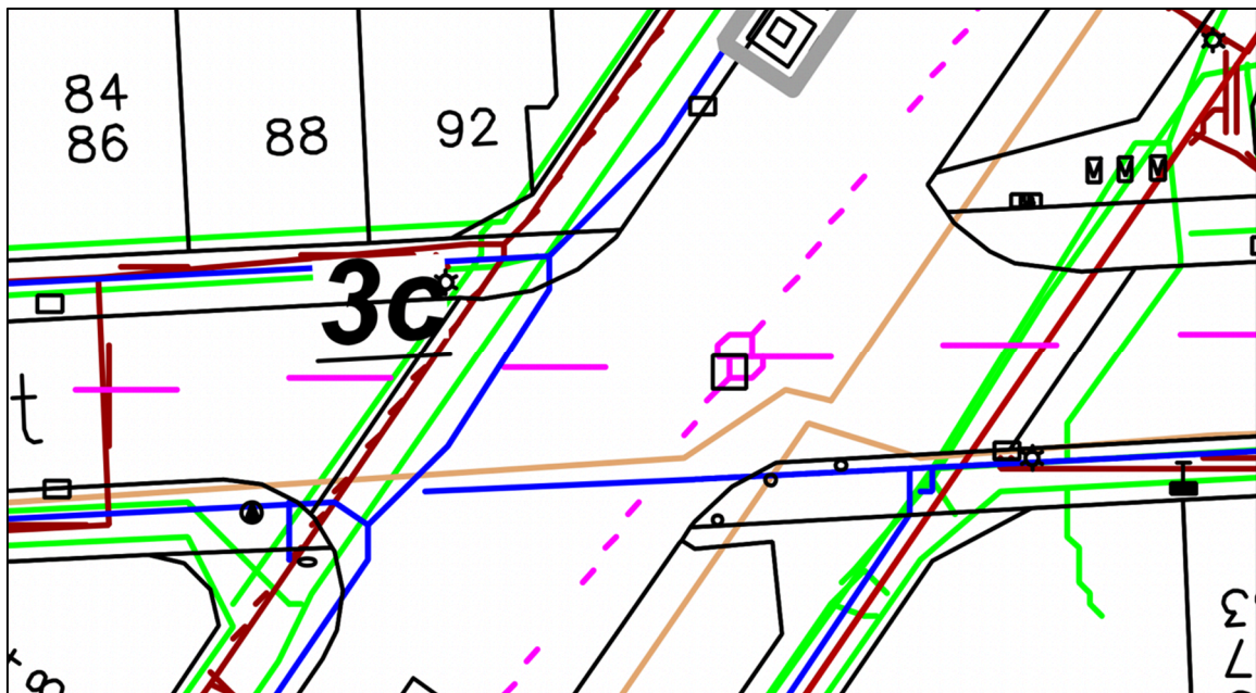
Afbeelding bij vraag 8: Kabels en leidingen in Douzastraat en Jan van Houtstraat. De lichtbruine lijnen zijn gasleidingen.
